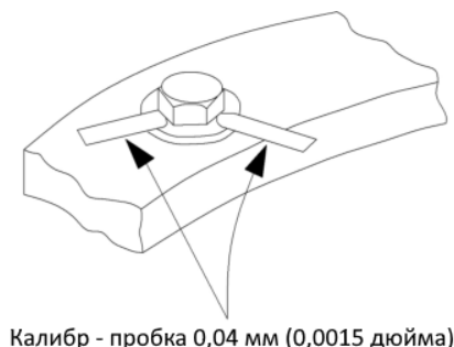
Калибр - пробка 0,04 мм (0,0015 дюйма)
